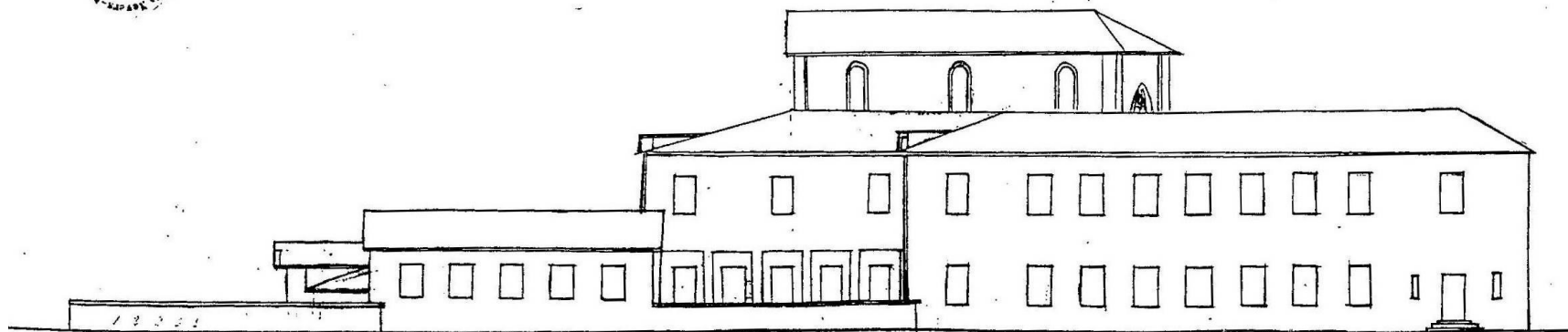
Facade Latérale
