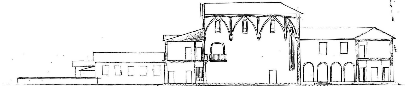
Croquis Longitudinal
